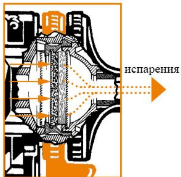
Рабочая камера наполнена не полностью, но сверху находится подушечка для маслянистых жидкостей
