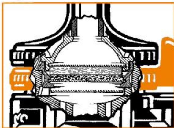
Рабочая камера наполнена не полностью, но сверху находится подушечка для маслянистых жидкостей
